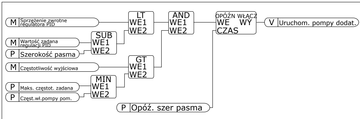
Rys. 101: Częst.wł.pompy pom.
