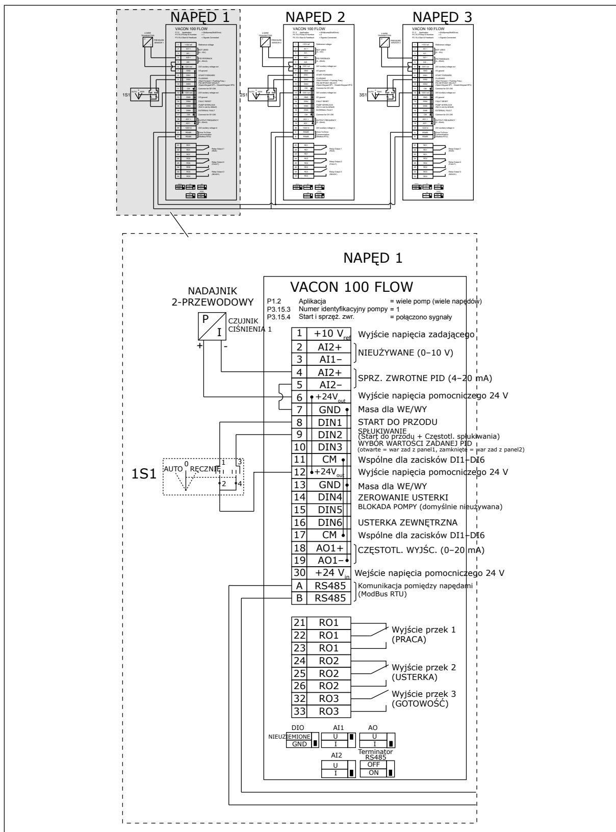
Rys. 18: Schemat połączeń elektrycznych w systemie wielonapędowym (wielonapędowym), przykład 1A
