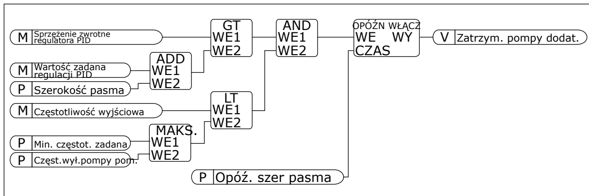
Rys. 102: Czest.wył.pompy pom.
