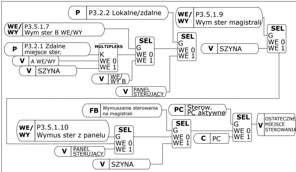
Rys. 41: Miejsce sterowania
