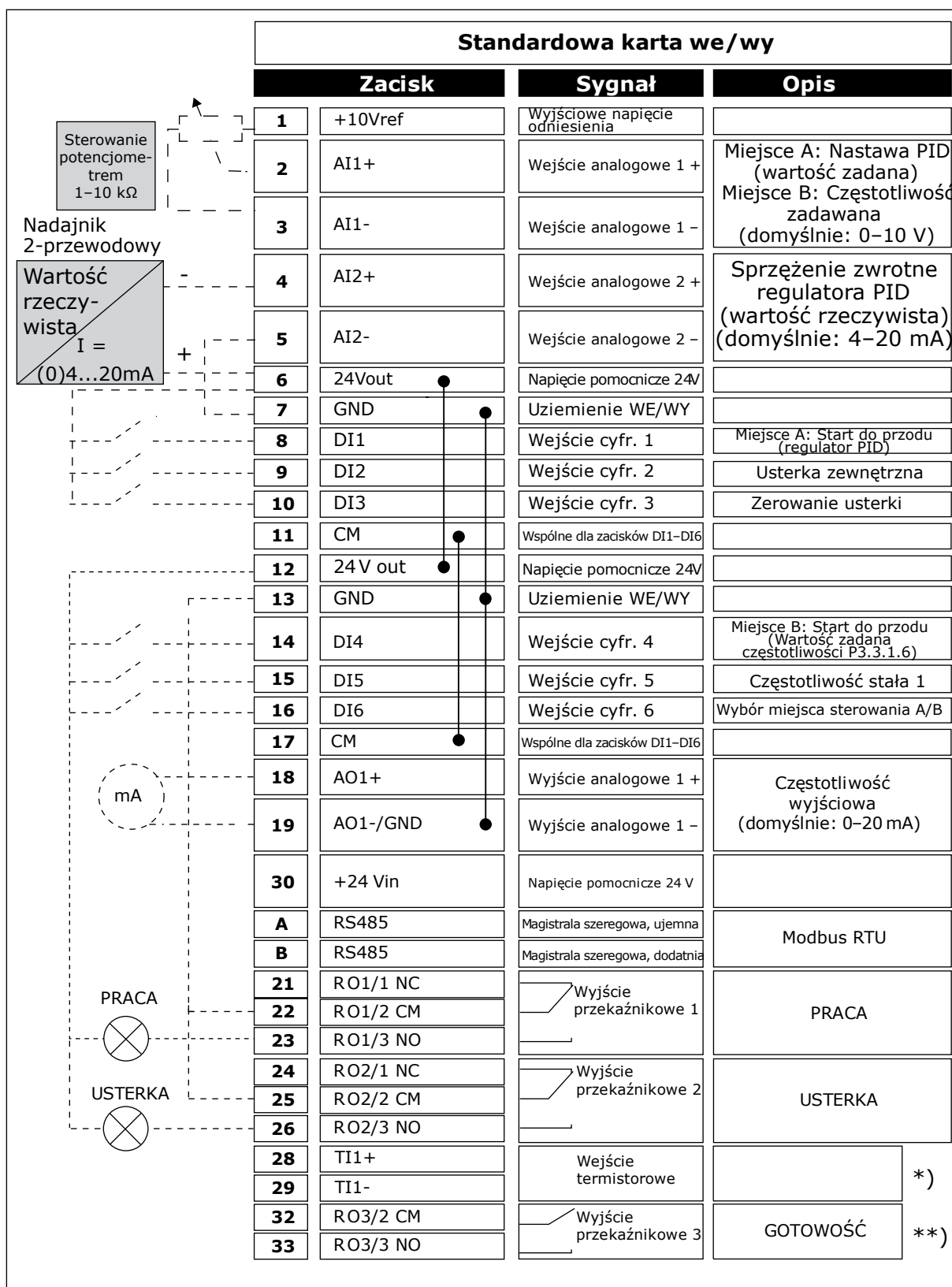
Rys. 6: Domyślne podłączenia sterowania aplikacji sterowania PID
