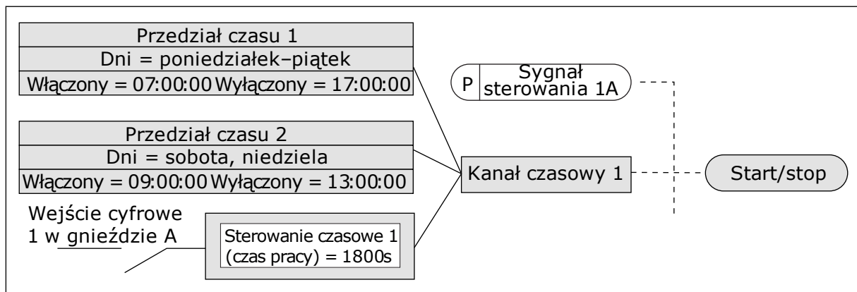
Rys. 78: Sygnał sterujący dla polecenia startu pochodzi z kanału czasowego 1, a nie z wejścia cyfrowego
